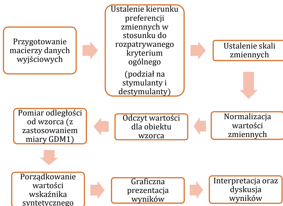
Ryc. 29. Uproszczony schemat procedury porządkowania liniowego z użyciem uogólnionej miary odległości GDM1
